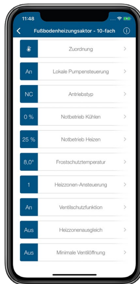
Abbildung 34: Screenshots Konfiguration HmIP-FAL-xx zur Pumpensteuerung
