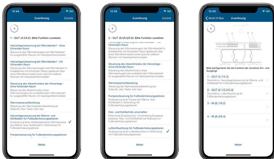
Abbildung 33: Screenshot Konf. HmIP-MIOB zur Steuerung von Pumpen/Heizkesseln/Luftentfeuchtern
