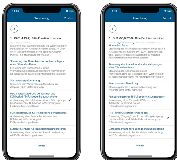
Abbildung 42: Screenshot Konfiguration Multi IO Box für Feuchtebegrenzer (1)
