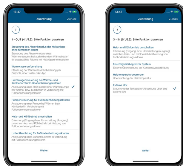
Abbildung 49: Screenshot Konfiguration Externe Schaltuhr (HmIP-MIOB)
