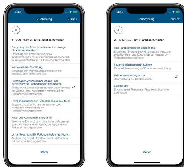
Abbildung 46: Screenshot Konfiguration HmIP-MIOB für Temperaturbegrenzung
