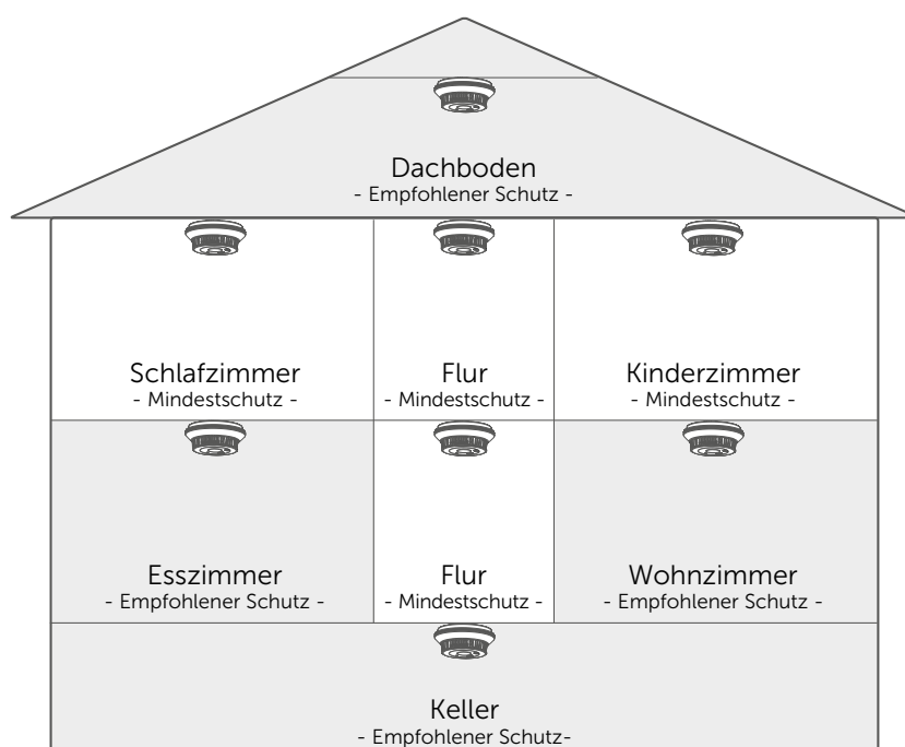
Abbildung 54: Installationshinweise Homematic IP Rauchwarnmelder mit Q-Label
