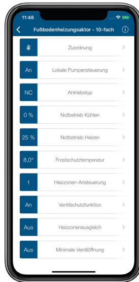
Abbildung 29: Screenshots Konfiguration HmIP-FAL-xx zur Pumpensteuerung
