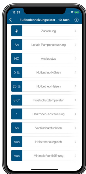
Abbildung 41: Screenshots Konfiguration HmIP-FAL-xx
