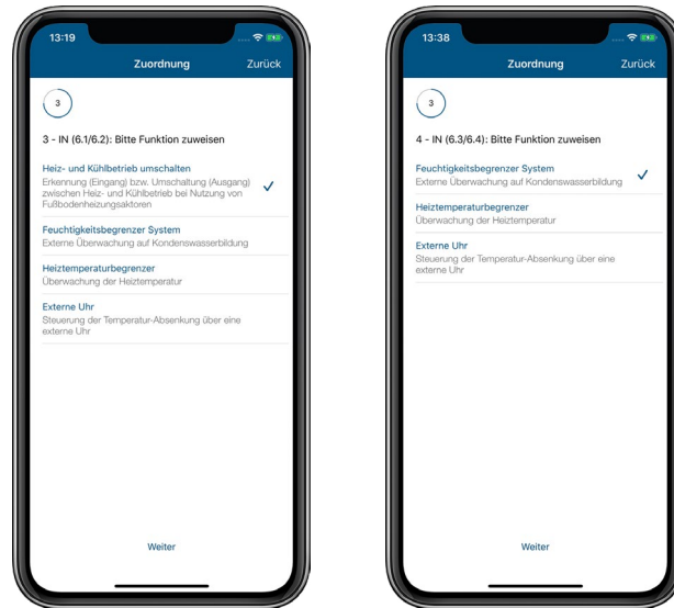
Abbildung 43: Screenshot Konfiguration Multi IO Box für Feuchtebegrenzer (2)
