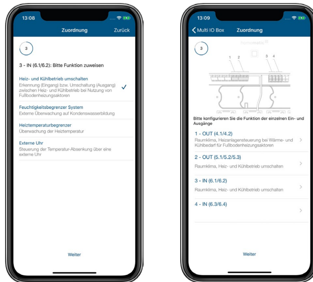
Abbildung 40: Screenshot Konfiguration Multi IO Box für Wechsel zwischen Heiz- und Kühlbetrieb über einen extern angeschlossenen Schalter (2)
